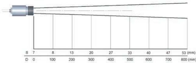
15:1 Optik
