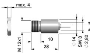
Messkopf
